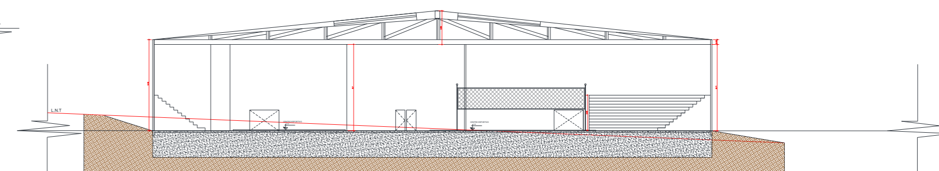
Corte Transversal DD
